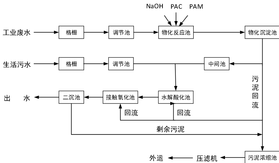
图 2 园区污水厂污水处理工艺流程图
